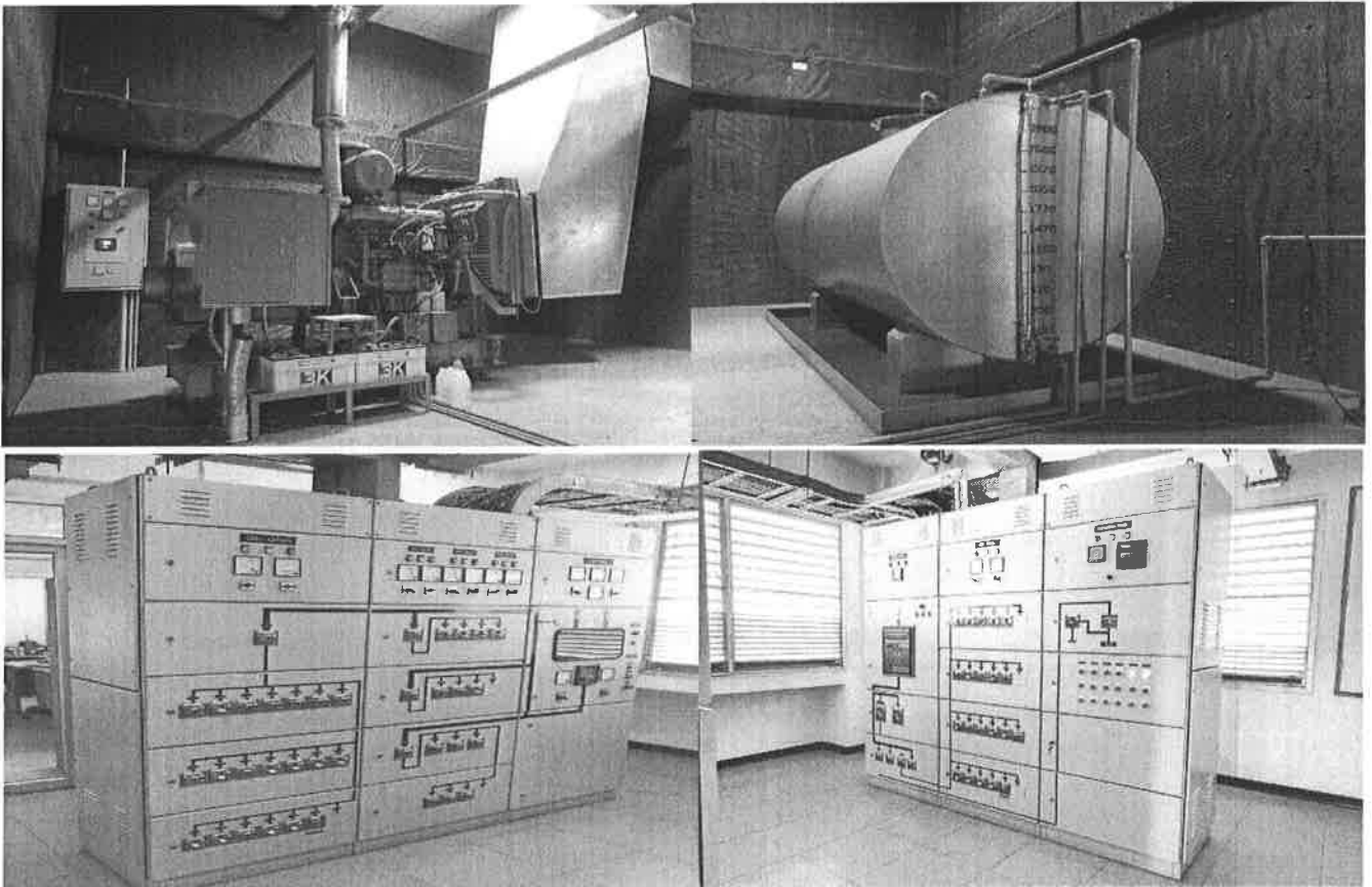
เครื่องตัดสลับไฟอัตโนมัติ (ATS)/เครื่องกำเนิดไฟฟ้าและวัสดุทั่วไป
