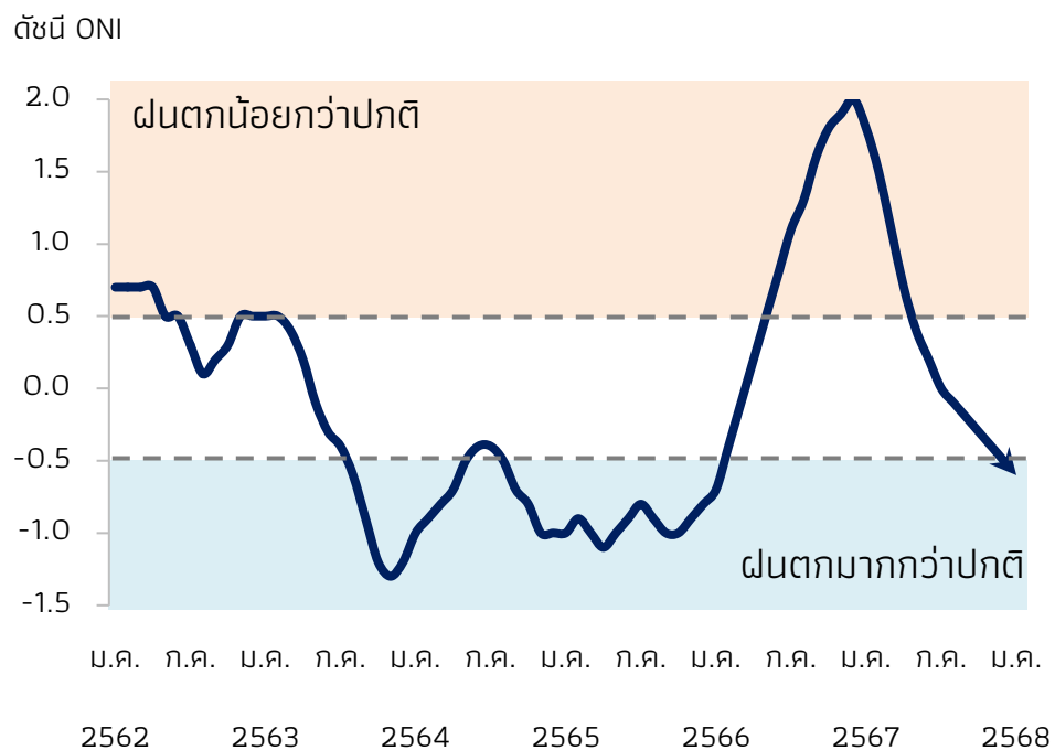
ดัชนี Oceanic Niño Index (ONI)
